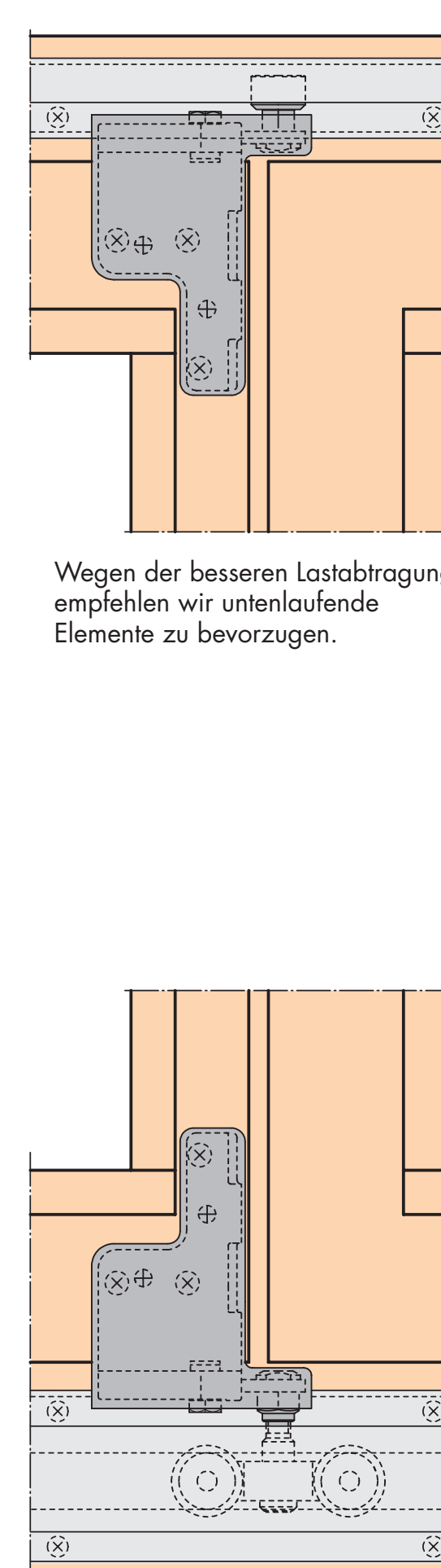
Schnittpunkt untenlaufend 1:2,5
